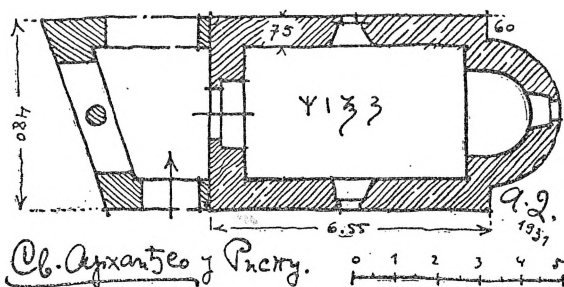
Сл. 5. — Основа црквице Св. Арханђела у Рисну.
