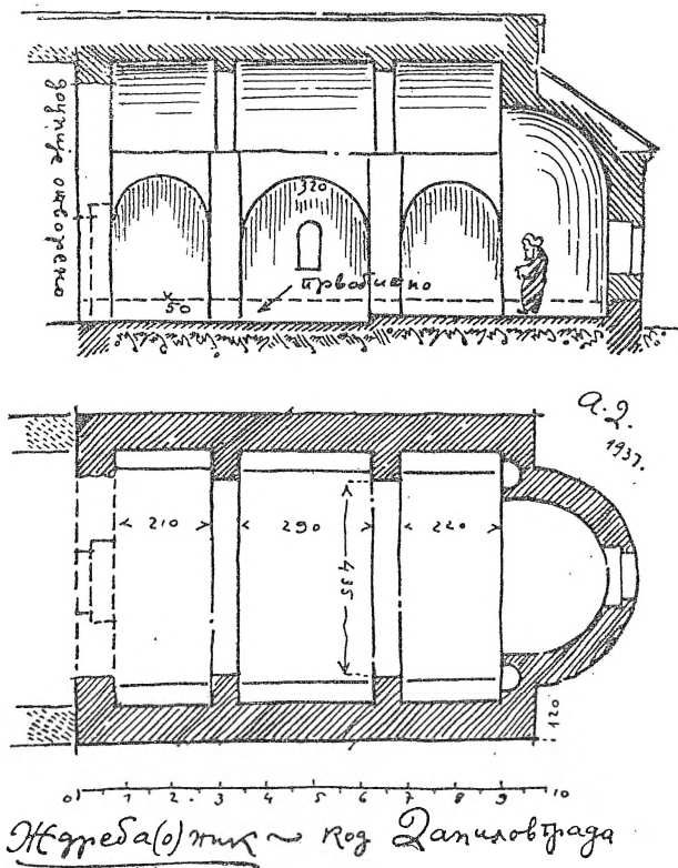
Сл. 1. — Основа и пресек цркве манастира Ждребаоника код Даниловграда у Црној Гори.
