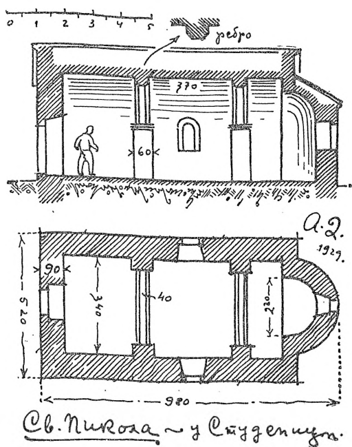
Сл. 6. — Основа и пресек црквице Св. Николе у Студеници.
