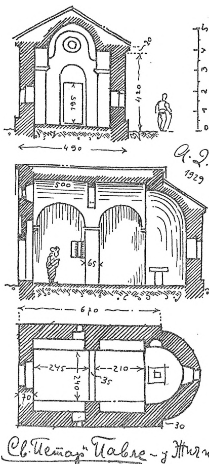
Сл. 8. — Основа и пресеци црквице Св. Петра и Павла у манастиру Жичи,
